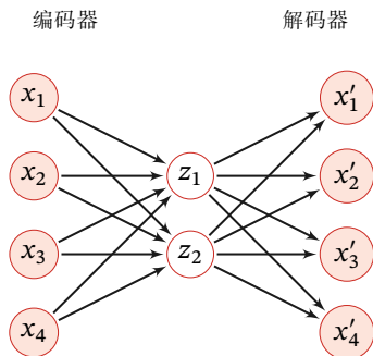
图 9.2 两层网络结构的自编码器
