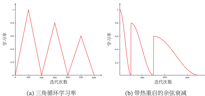
图 7.5 周期性学习率调整
