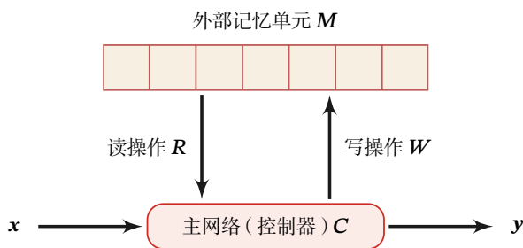
图 8.6 记忆网络的典型结构
