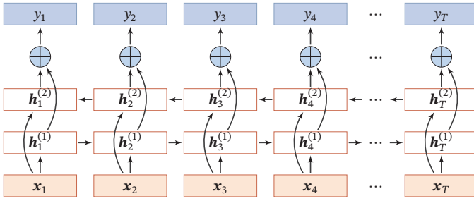
图 6.10 按时间展开的双向循环神经网络
