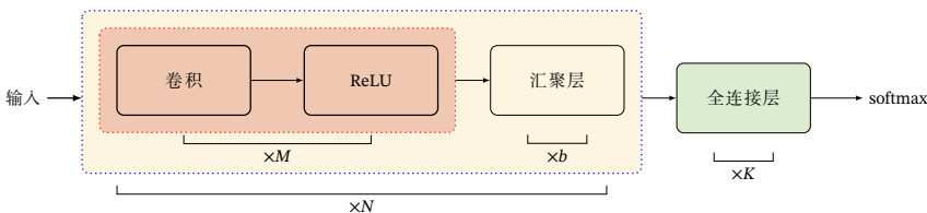
图 5.9 典型的卷积网络结构
