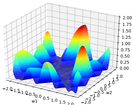
图 7.2 神经网络中的平坦底部示例
