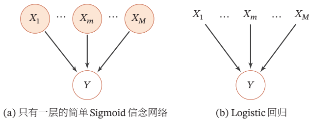
图 11.4 Sigmoid 信念网络和 Logistic 回归模型比较
