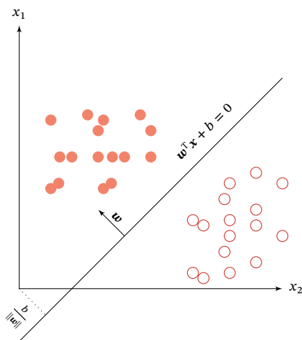
图 3.2 二分类的决策边界示例
