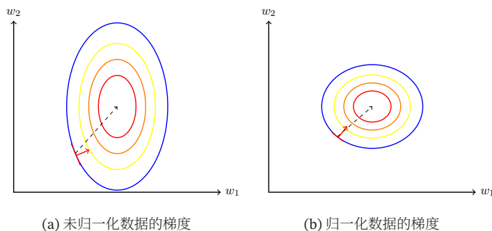
图 7.9 数据归一化对梯度的影响
