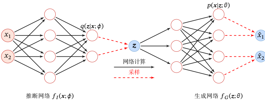
图 13.4 变分自编码器的网络结构
