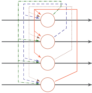
图 8.10 四个节点的 Hopfield 网络
