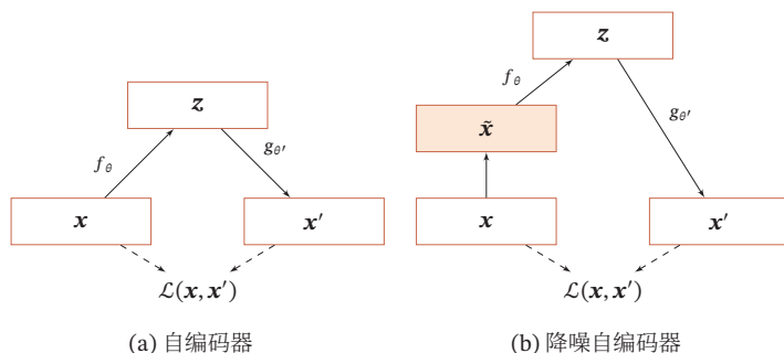
图 9.3 自编码器和降噪自编码器
