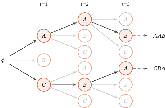
图 15.1 束搜索过程示例
