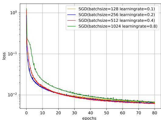
(b) 按 Epoch 的损失变化
