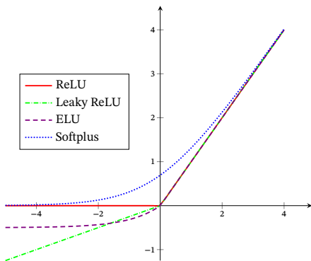
图 4.4 ReLU、Leaky ReLU、ELU 以及 Softplus 函数
