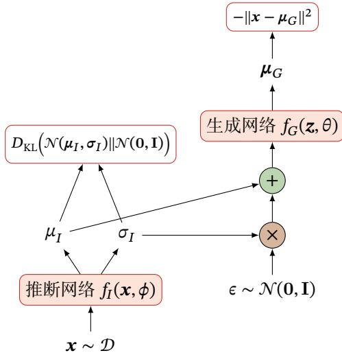
图 13.5 变分自编码器的训练过程
