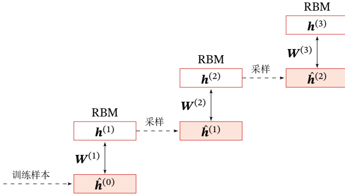
图 12.6 深度信念网络的逐层预训练过程
