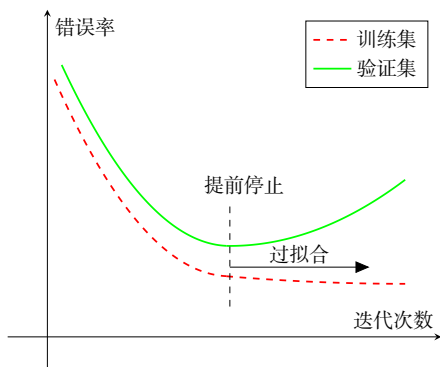
图 2.4 提前停止示例
