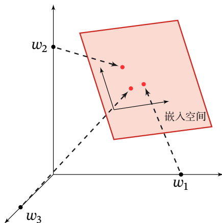
图 1.3 one-hot 向量空间与嵌入空间
