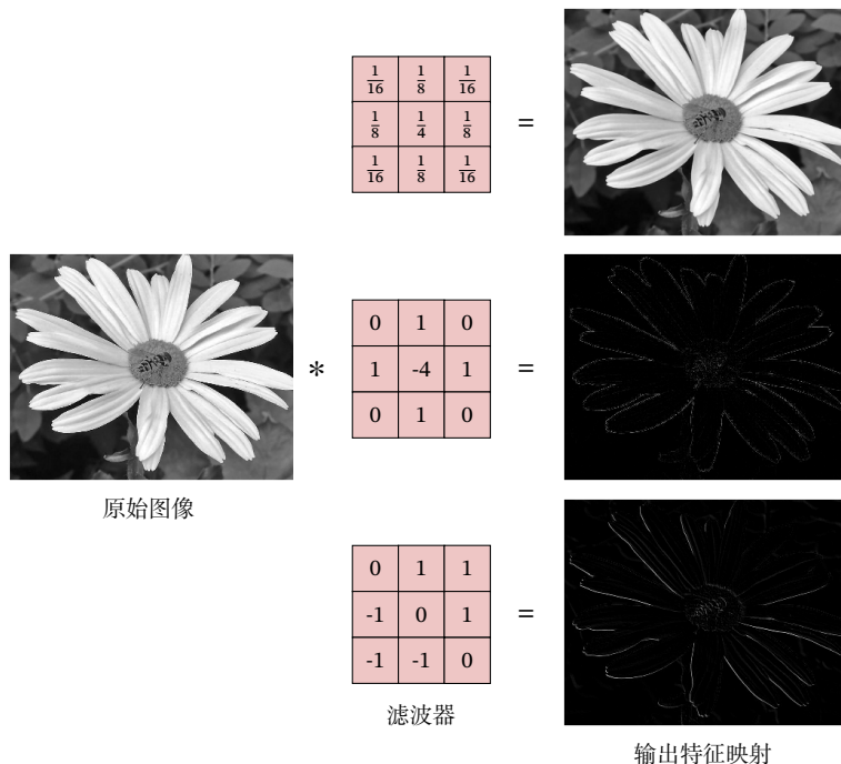
图 5.3 图像处理中几种常用的滤波器示例
