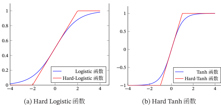
图 4.3 Hard Sigmoid 型激活函数
