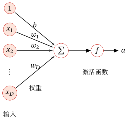
图 4.1 典型的神经元结构
