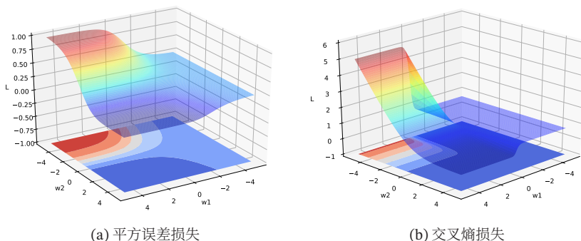
图 4.10 神经网络 y = \sigma(w_2 \sigma(w_1 x)) 的损失函数
