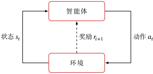
图 14.2 智能体与环境的交互
