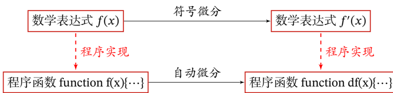
图 4.9 符号微分与自动微分对比
