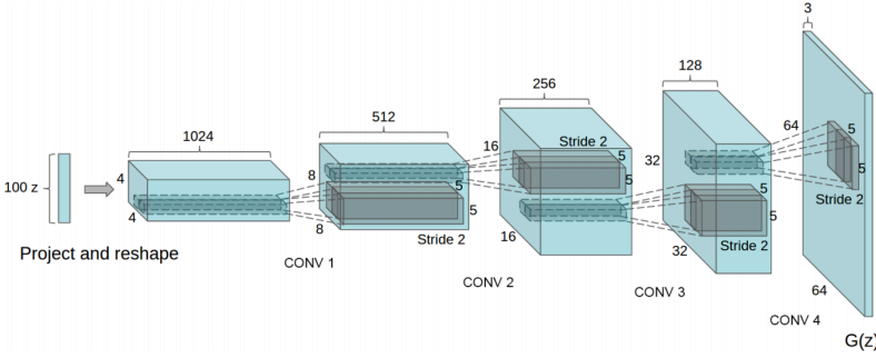
图 13.9 DCGAN 中的生成网络. 第一层是全连接层, 输入是从均匀分布中随机采样的 100 维向量 \mathbf{z} , 输出是 4 \times 4 \times 1024 的向量, 重塑为 4 \times 4 \times 1024 的张量; 然后是四层的微步卷积, 没有汇聚层. 图片来源: [Radford et al., 2016]
