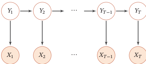
图 11.6 隐马尔可夫模型
