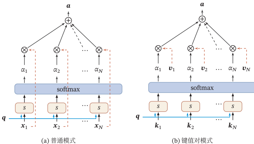
图 8.1 注意力机制
