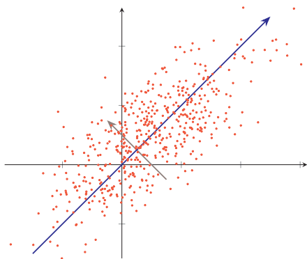
图 9.1 主成分分析
