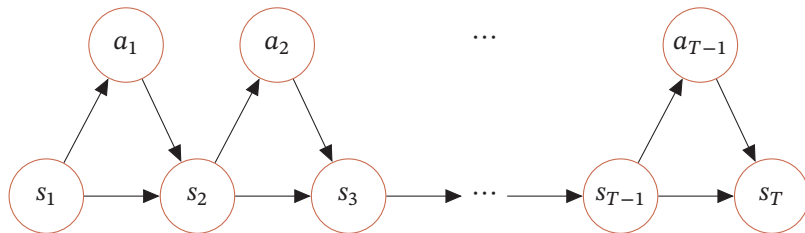
图 14.3 马尔可夫决策过程
