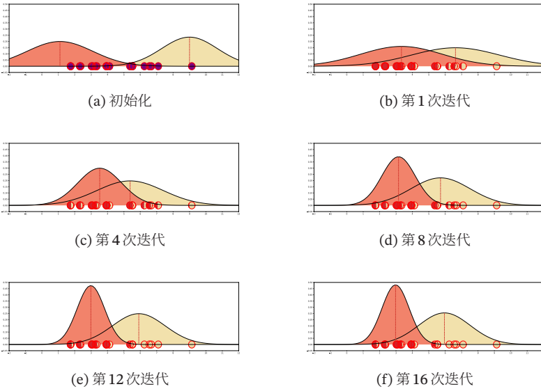
图 11.13 高斯混合模型训练过程示例
