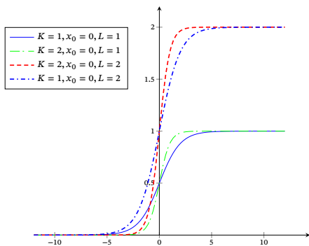
图 B.3 Logistic 函数
