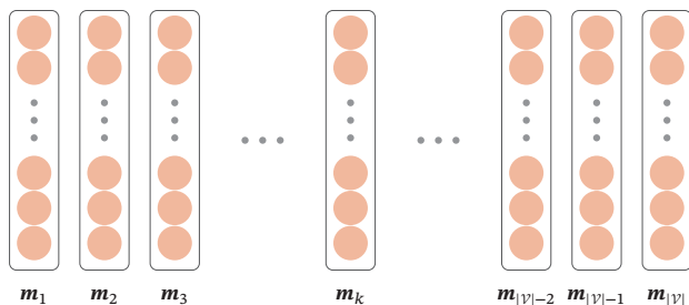
图 15.2 嵌入矩阵
