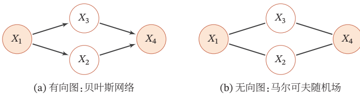
图 11.2 有向图和无向图示例
