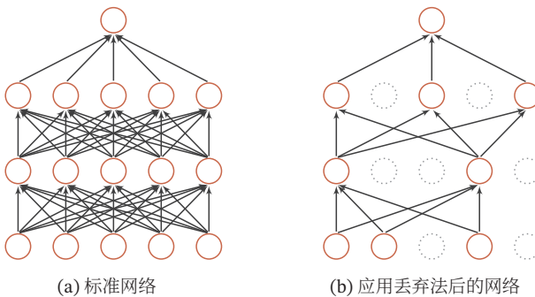
图 7.12 丢弃法示例
