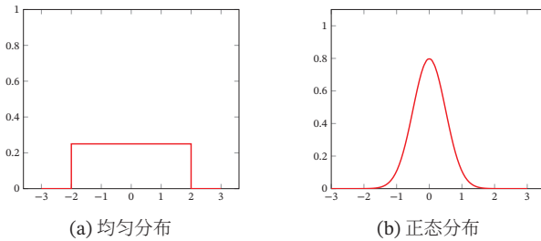
图 D.1 连续随机变量的密度函数
