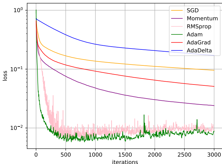
图 7.8 不同优化方法的比较
