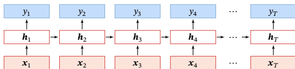
图 6.2 按时间展开的循环神经网络
