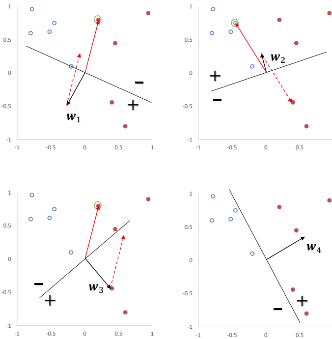
图 3.5 感知器参数学习的更新过程
