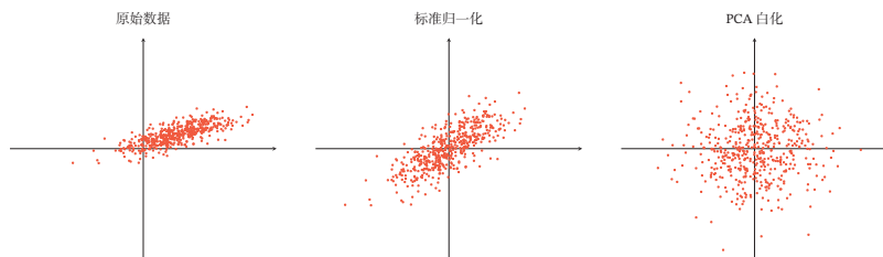
图 7.10 标准归一化和 PCA 白化
