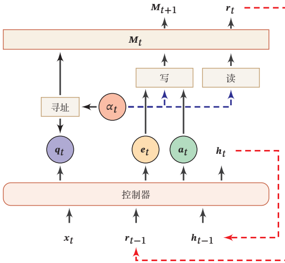
图 8.9 神经图灵机示例
