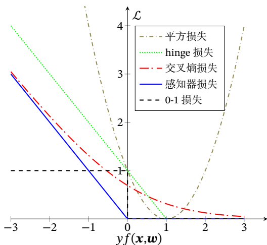
图 3.7 不同损失函数的对比
