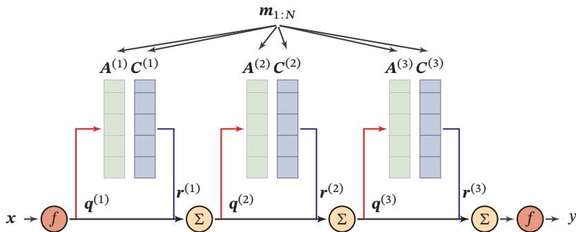
图 8.7 端到端记忆网络
