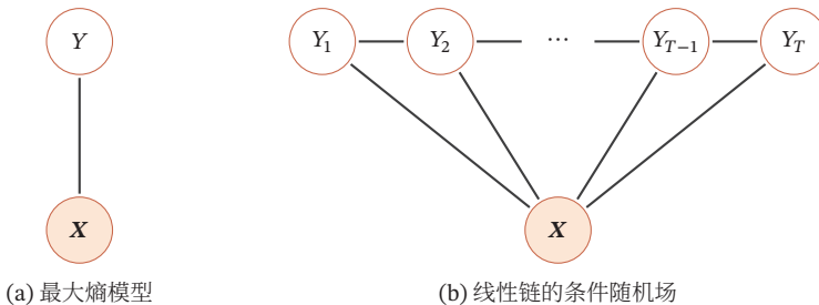
图 11.8 最大熵模型和线性链条件随机场
