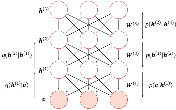
图 12.5 一个有 4 层结构的深度信念网络
