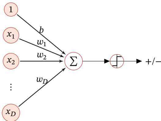
图 3.1 二分类的线性模型
