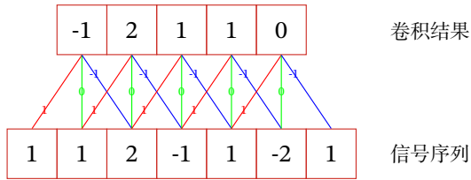
图 5.1 一维卷积示例 (滤波器为 [-1, 0, 1] )
