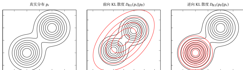
图 13.11 前向和逆向 KL 散度
