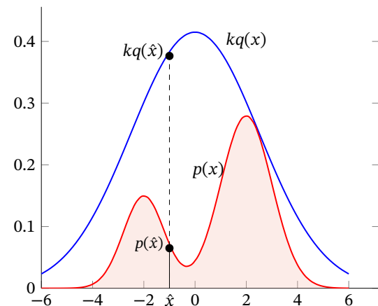
图 11.15 拒绝采样
