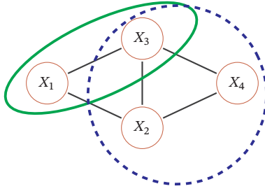
图 11.7 无向图模型中的团和最大团
