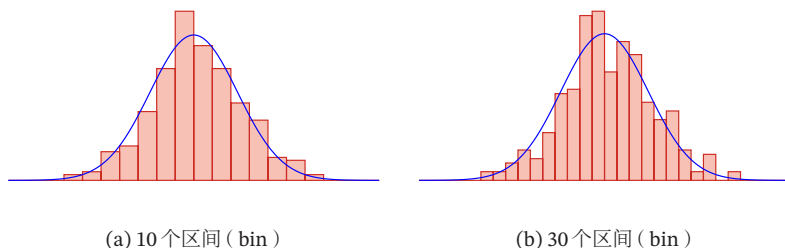
图 9.4 直方图密度估计
