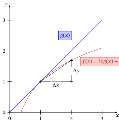
图 B.1 函数 f(x) = \log(x) + 1 的导数
