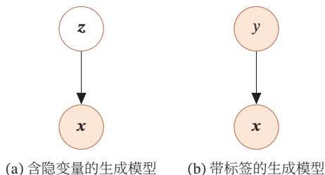
图 13.2 生成模型
