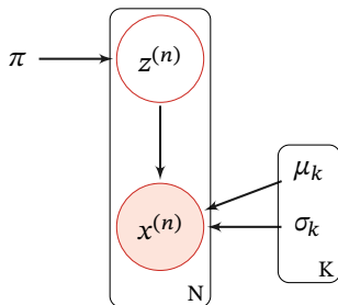
图 11.12 高斯混合模型
