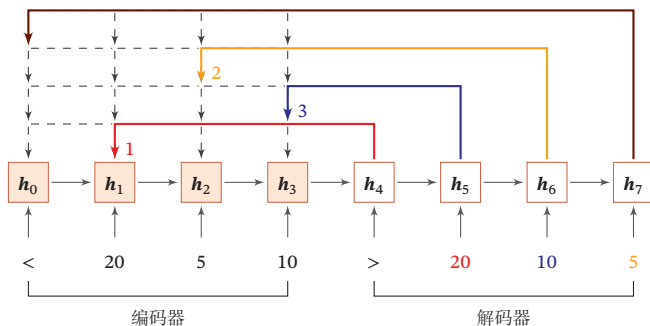
图 8.2 指针网络
