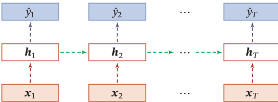
图 7.14 变分丢弃法
