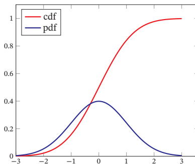
图 D.2 标准正态分布的概率密度函数和累积分布函数
