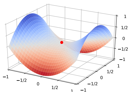
图 7.1 鞍点示例
