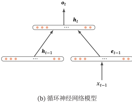
图 15.3 深度序列模型
