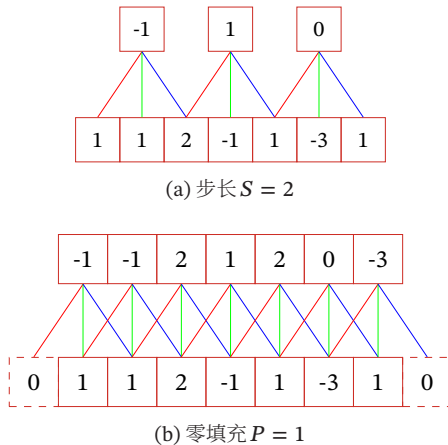
图 5.4 卷积的步长和零填充
