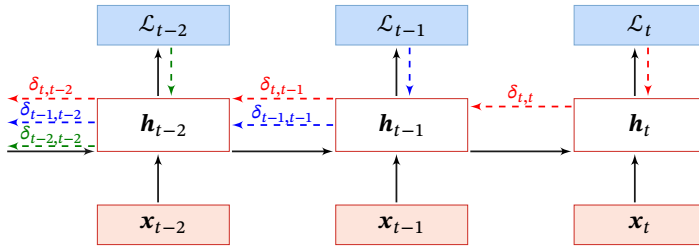
图 6.6 误差项随时间反向传播算法示例
